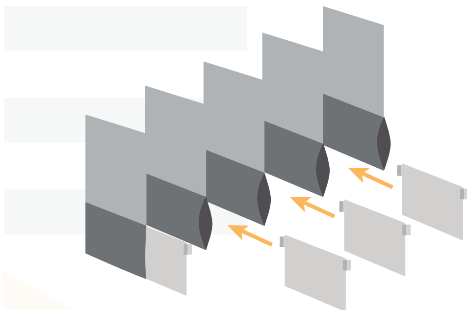
Colocação de contrapesos
